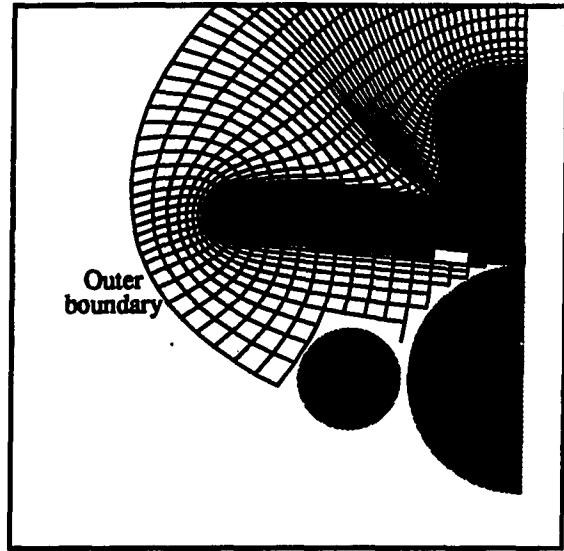
(b) ORB grid
